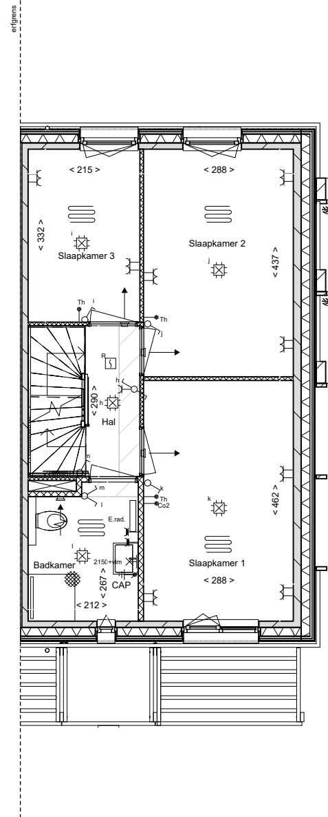
eerste verdieping
