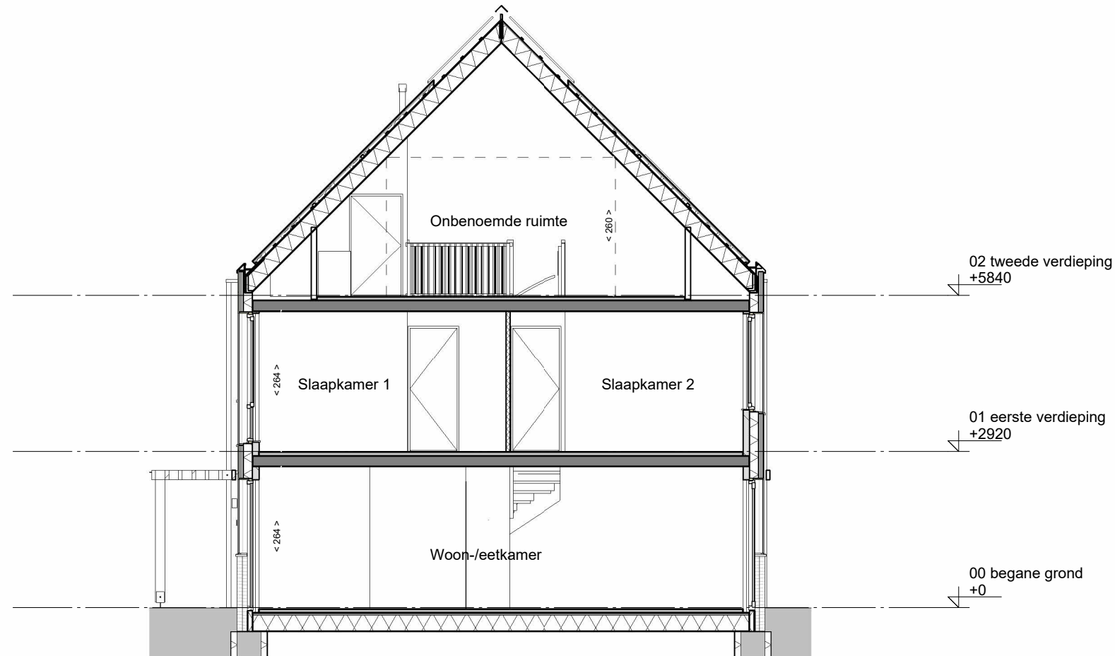
doorsnede
