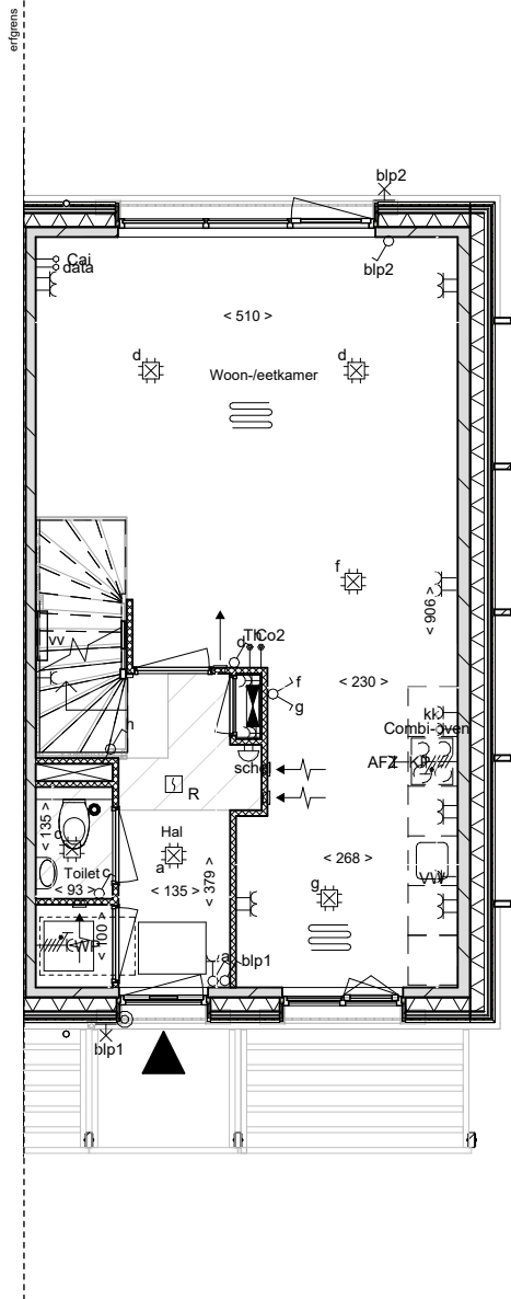
begane grond
